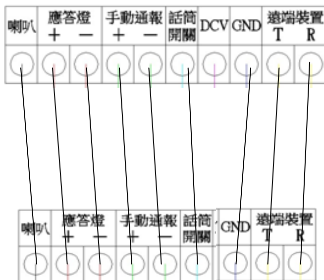
119 電源增設裝置(左邊端子座上/下層) ↑
