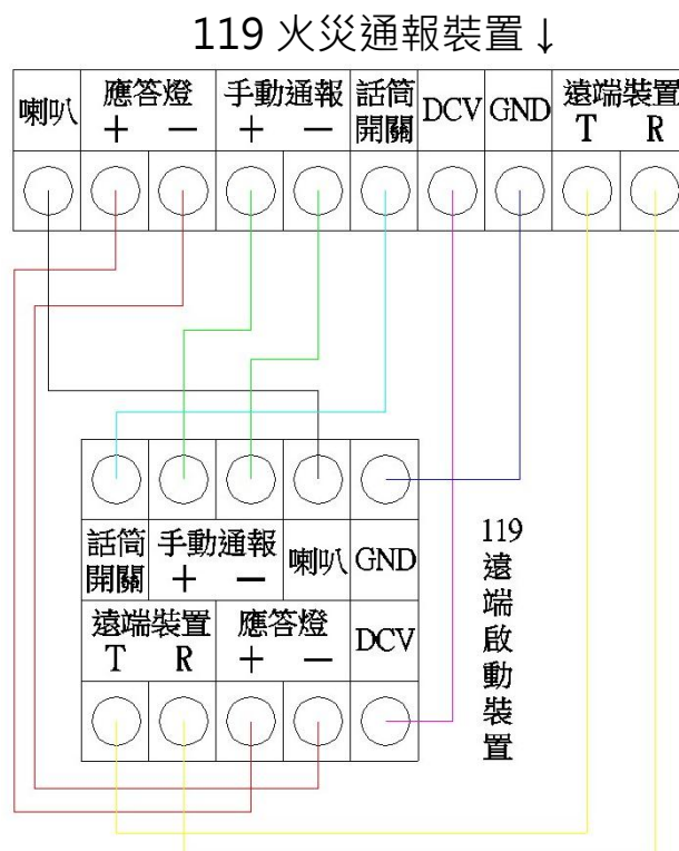
本機+119 遠端啟動裝置(Max:4 具) 配線詳圖
