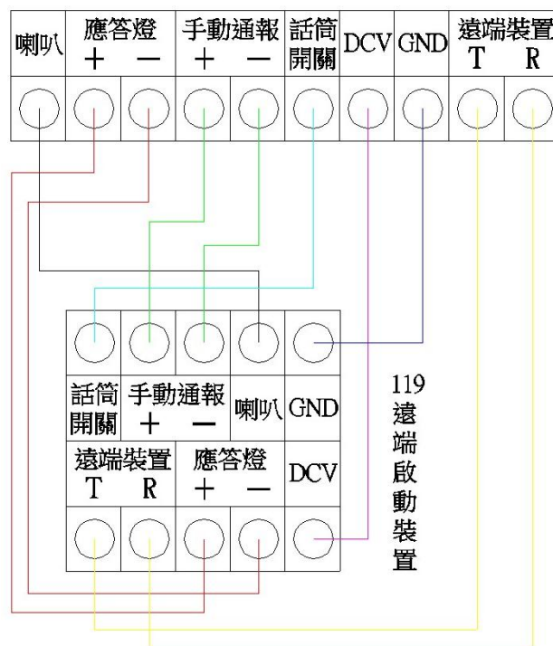
119 電源增設裝置右邊下層端子: ↓ (可連接 4 具 119 遠端啟動裝置)
