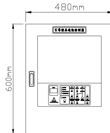
外部配置圖
