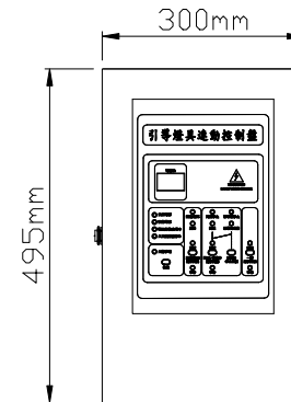
外部配置圖
