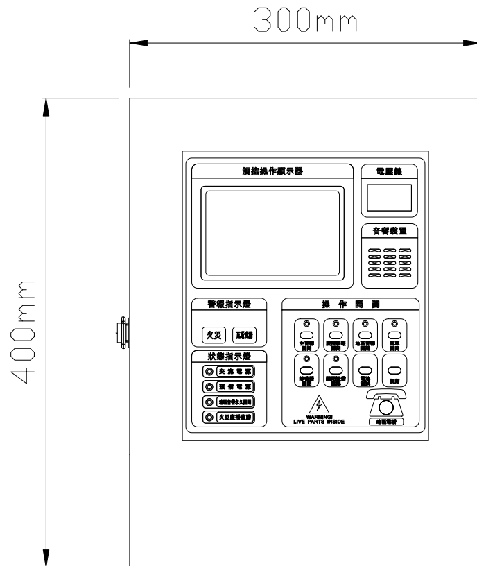
外部配置圖
