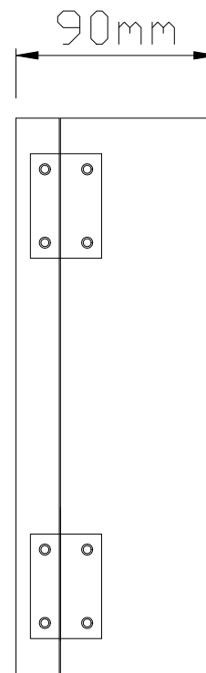
側視圖
