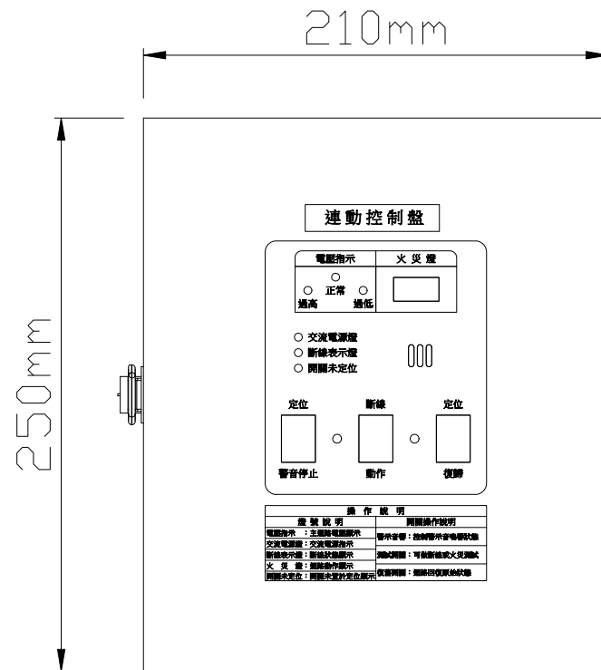
外部配置圖
