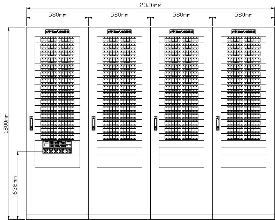
外部配置圖
