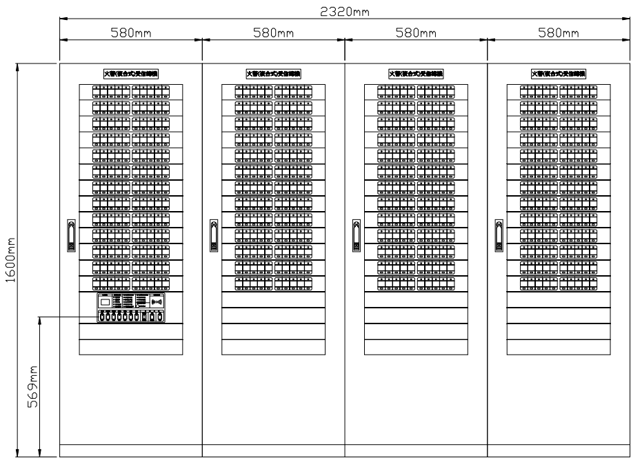
外部配置圖
