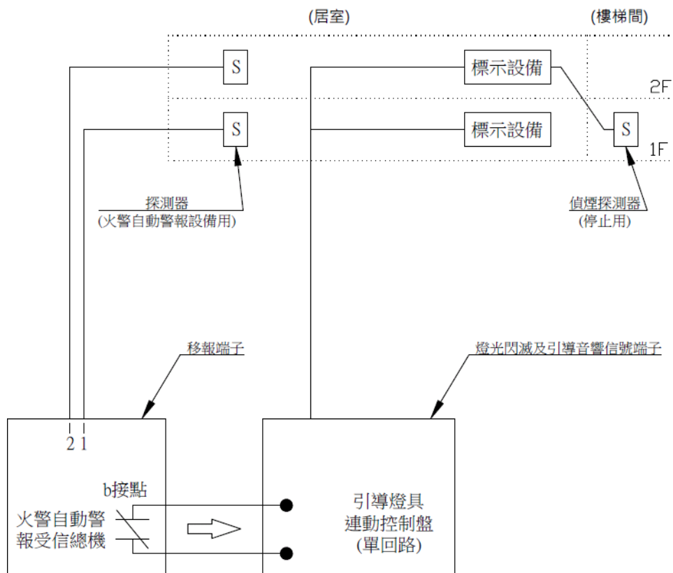
YLP-PO_配線圖
